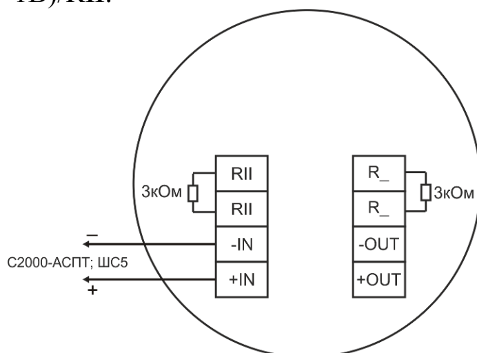
Рисунок 5 – Схема подключения УДП к С2000-АСПТ
