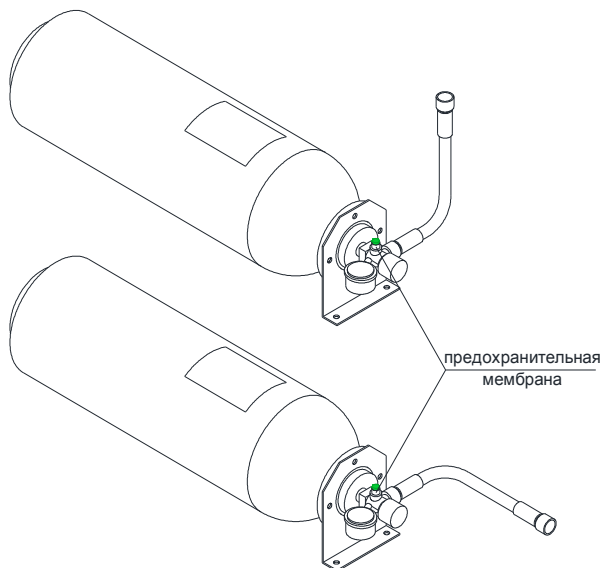
Рисунок 7 - Модуль МПТХ (150-20/32-12)-Г. Пример монтажа.
